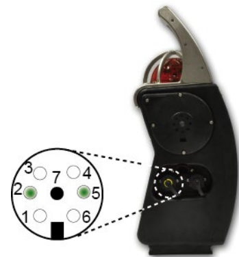
Figure 7 : entrées logiques.
