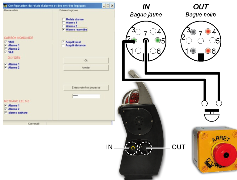
Figure 12 : Connexion d'un bouton coup de poing sur une balise (exemple). Se référer au chapitre L'application COM 2100 , en page 37, pour le paramétrage
