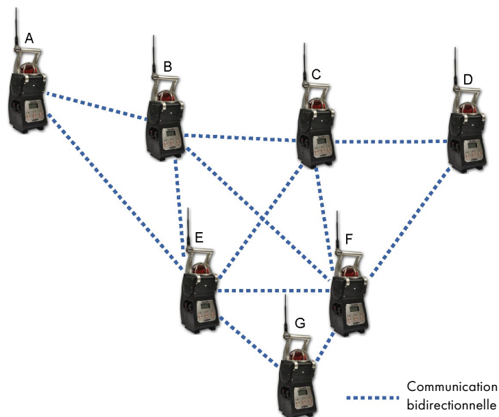
Figure 21 : dans cet exemple, la BM 25AW G communique avec E et F. Si la communication entre G et F est coupée, E continue d'assurer la liaison. Si G part en alarme ou en défaut, toutes les BM 25AW du réseau indiqueront à leur tour une information d'alarme ou de défaut
