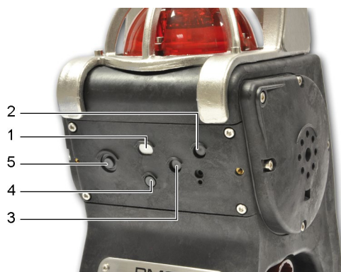
Figure 8 : position des cellules
