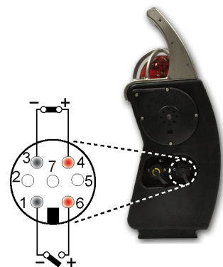
Figure 6 : sorties des relais
