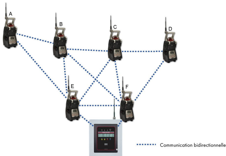
Figure 24 : dans cet exemple, les BM 25AW E et F sont les derniers maillons entre le réseau de balises et le système de centralisation. Si la communication entre la MX 40 et la BM 25AW F est coupée, E continue d'assurer la liaison. Si A part en alarme gaz ou en défaut, la centrale reçoit l'information et répercute l'information d'alarme gaz sur toutes les balises (selon programmation).
