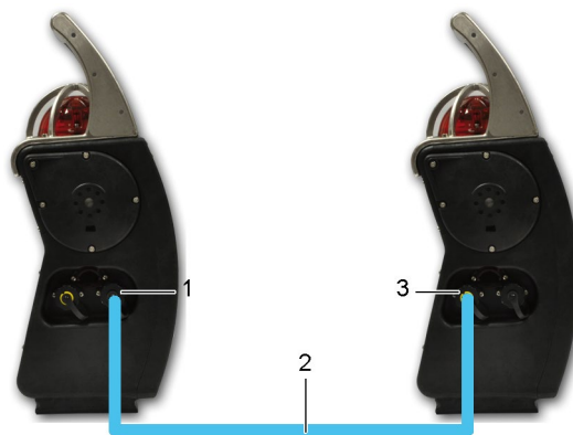
Figure 18 : liaison inter-balises
