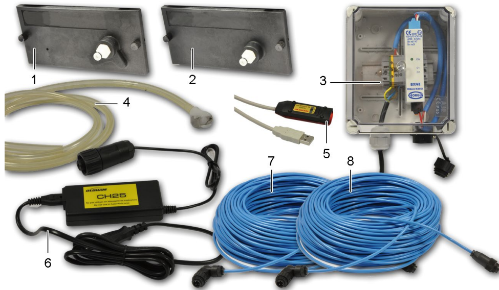
Figure 3 : les accessoires
