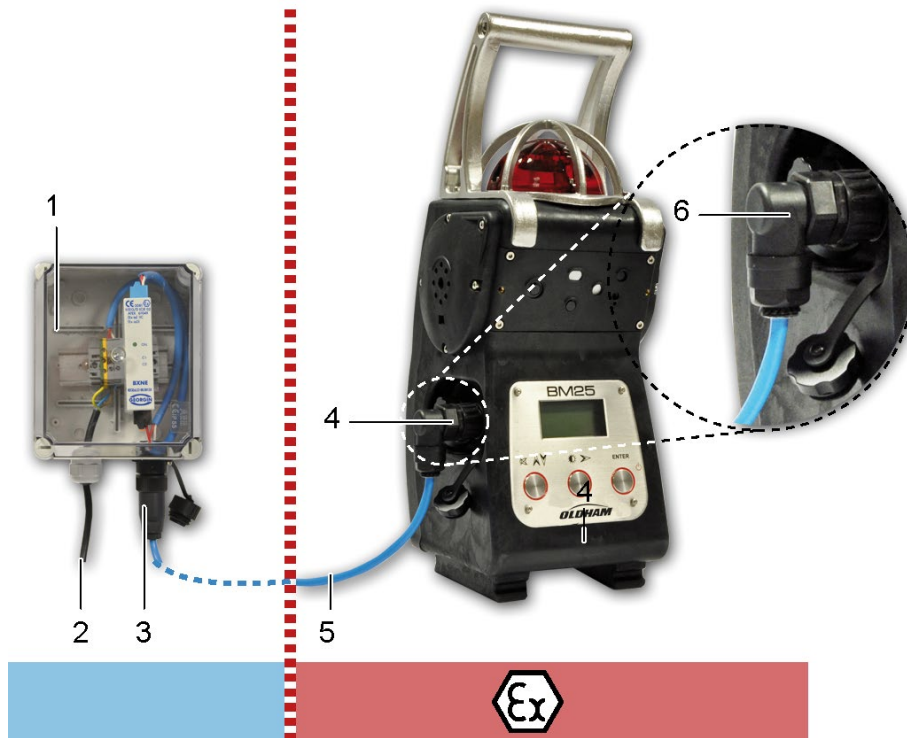
Figure 11 : Raccordement du dispositif de biberonnage
