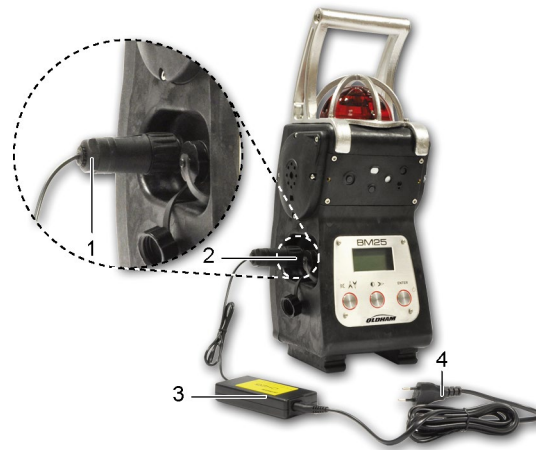
Figure 10 : charge en zone sûre
